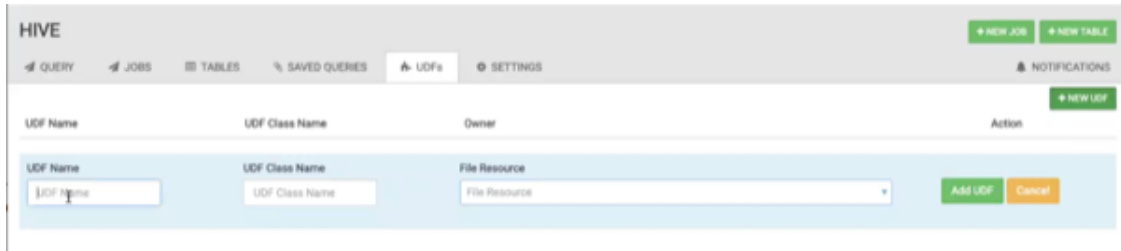
Figure 6.15. UDF Tab
